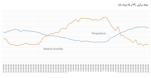
نمودار ۱۳- نمودار دما و رطوبت نسبی حیاط مرکزی در خردادماه (مأخذ: نگارنده)
