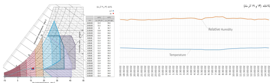
نمودار ۲۴- نمودار آذرماه زیست‌اقلیمی (گیوانی) بالاخانه (مأخذ: نگارنده)
