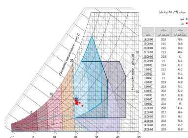
نمودار ۱۲- نمودار خردادماه زیست‌اقلیمی (گیوانی) سرداب (مأخذ: نگارنده)
