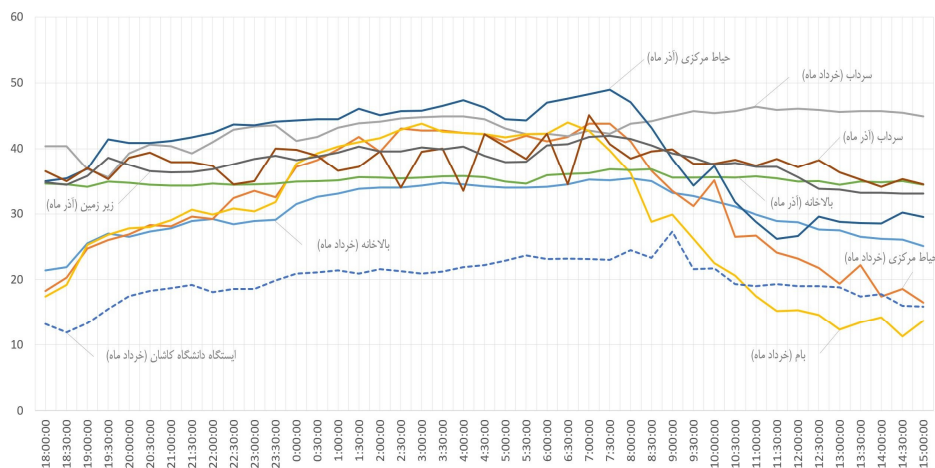
نمودار ۷- تغییرات رطوبت نسبی در خردادماه و آذرماه (مأخذ: نگارنده)
