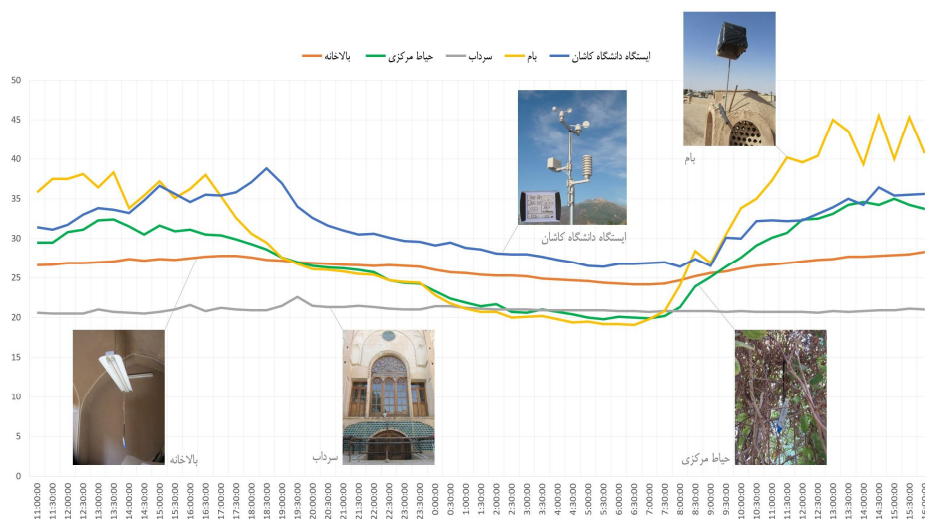
نمودار ۲- تغییرات دما در ۲۴ و ۲۵ خردادماه (مأخذ: نگارنده)
