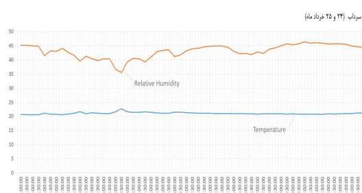
نمودار ۱۱- نمودار دما و رطوبت نسبی سرداب در خردادماه (مأخذ: نگارنده)
