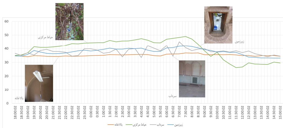
نمودار ۵- تغییرات رطوبت نسبی در ۱۸ و ۱۹ آذرماه (مأخذ: نگارنده)
