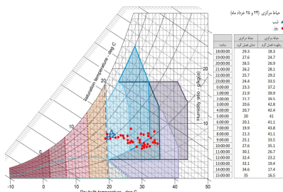
نمودار ۱۴- نمودار خردادماه زیست اقلیمی (گیوانی) حیاط مرکزی (مأخذ: نگارنده)
