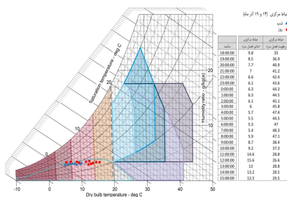
نمودار ۲۲- نمودار آذرماه زیست‌اقلیمی گیوانی (حیاط مرکزی (مأخذ: نگارنده)
