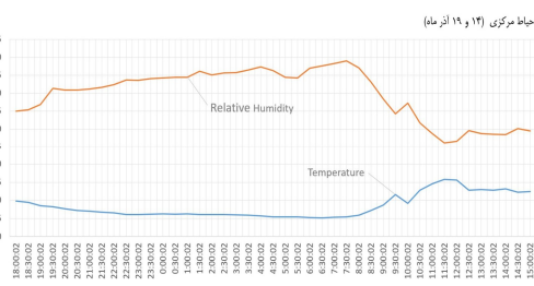
نمودار ۲۱- نمودار دما و رطوبت نسبی حیاط مرکزی در آذرماه (مأخذ: نگارنده)
